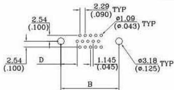
P.C.B LAYOUT (15Pins)
