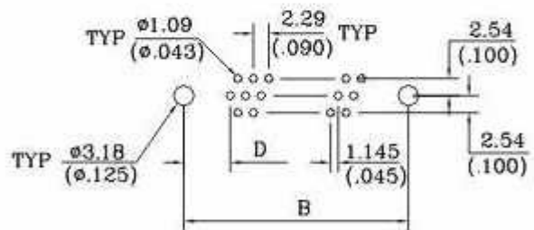
P.C.B LAYOUT(26,44,62Pins)
