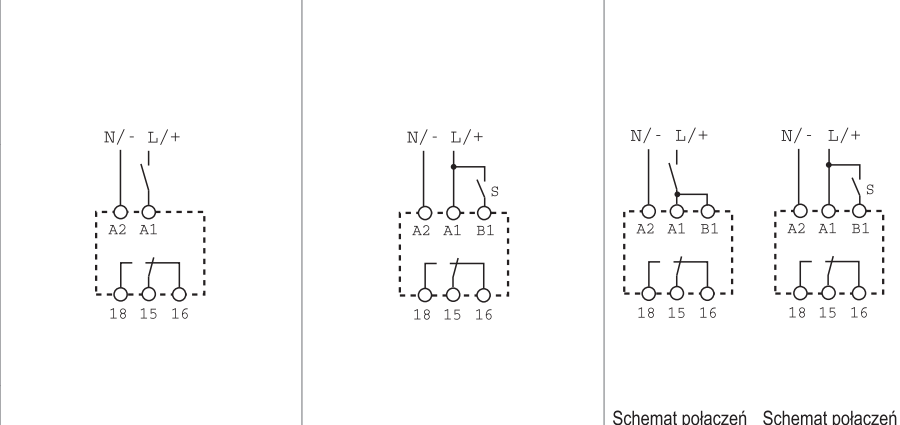
Schemat połączeń (bez sygnału START) Schemat połączeń (z sygnałem START) Schemat połączeń (bez sygnału START) Schemat połączeń (z sygnałem START)
