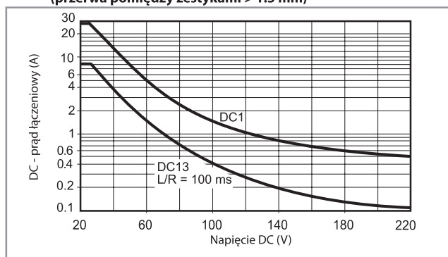
H 66 - Graniczna zdolność rozłączeniowa DC, wersja x60x (przerwa pomiędzy zestykami > 1.5 mm)
