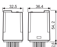
Typ 60.13/60.13 - 52xx
