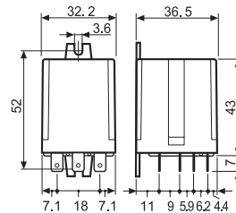
Typ 60.63
