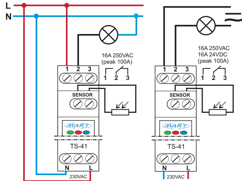
Rys. 2.: Schematy podłączenia AUTOMATU ZMIERZCHOWEGO TS-41-2.
