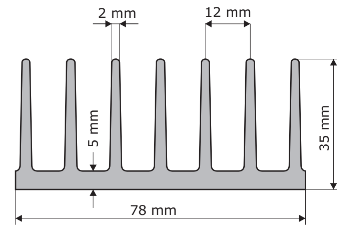
A5723 G=2,5 kg/m, P=9,65 cm 2 , O=56,46 cm
