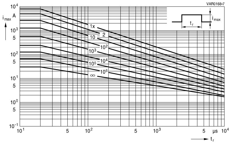
SIOV-S20K130 ... K320
