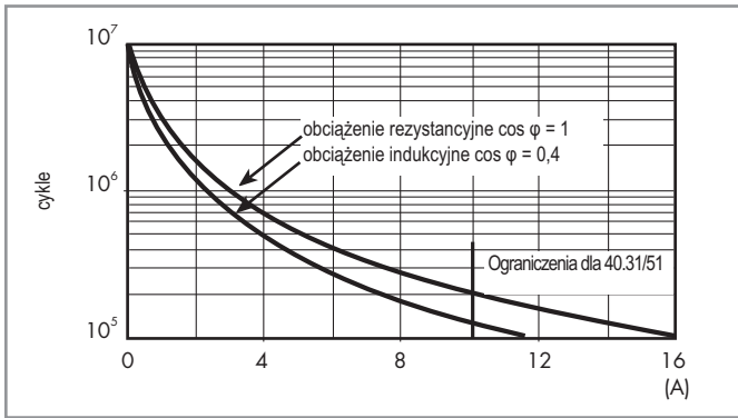
F 40 - Trwałość łączeniowa (dla AC) w funkcji prądu na zestykach Seria 40.31/51/61
