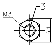
NUT t=2.3mm
