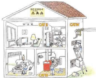
IEC 61010-1 标准规定的测量类别
